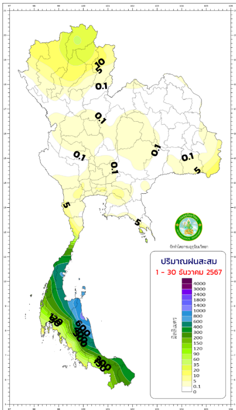
ปริมาณฝนสะสม 1-30 ธันวาคม 2567
